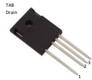
TO-247-4L
